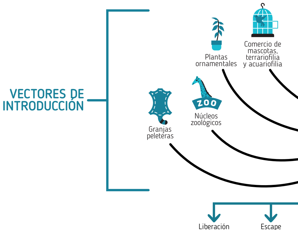
Figura 2. Principales vías de introducción y vías de entrada y dispersión de las especies invasoras.
